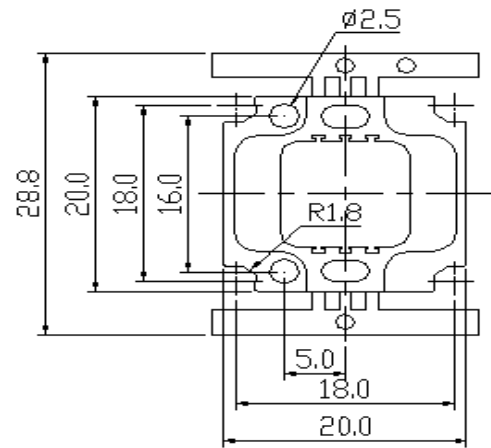
产品俯视图
