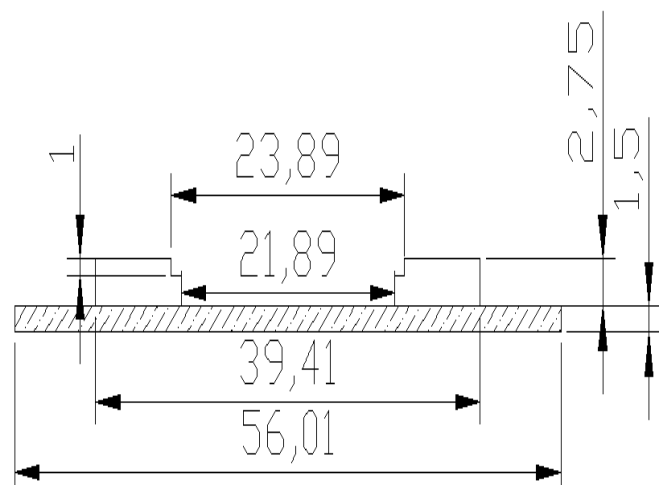
产品主视图
