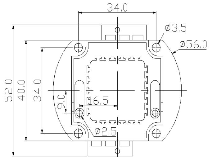
产品俯视图
